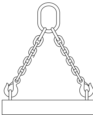
(d) Double-Leg Bridle Sling Hitch
