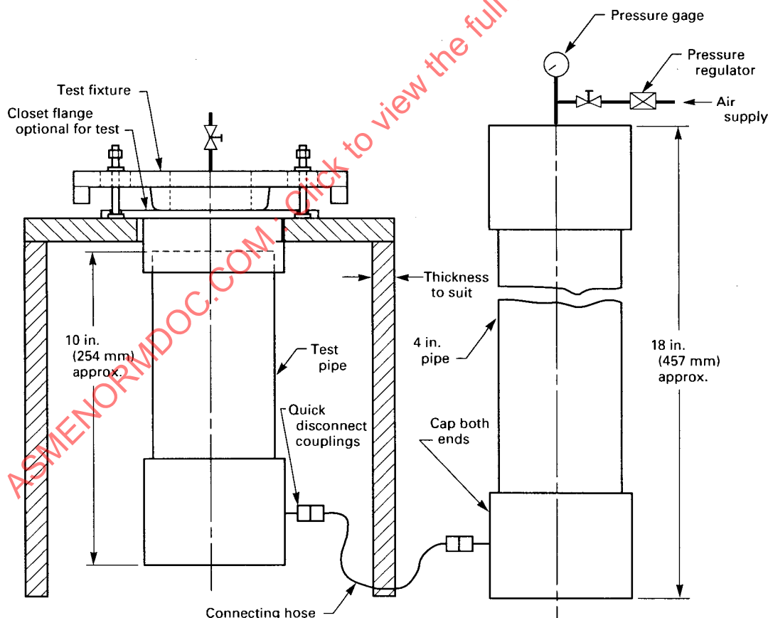
FIG. 1 TEST STAND
